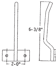
Hold Back Hook 515-9-78B
