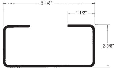
10 Ga. Steel x 106-1/4" 511-23-183-0-108
