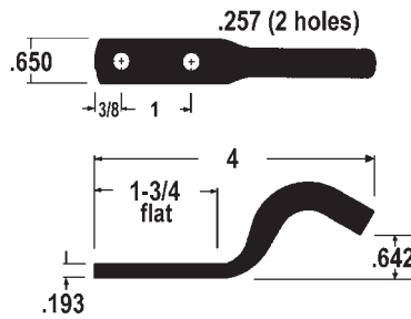
Hold Back Hook 515-9-81
