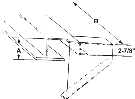
512-A8-156B A = 4-1/4"; B = 102-3/8"
