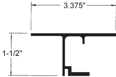
Trailmobile Reeper 90-4-1892-0-115 115" Aluminum
