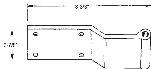
Door Hinge 516-2-47 Aluminum
