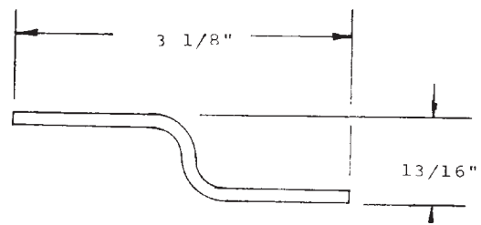
519-3-418-0-FO 103" 12 Ga. Steel
