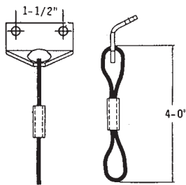
Hold Back Loop 515-9-78A
